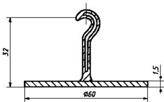
Черт.2. Верхняя стеклянная тарелка
