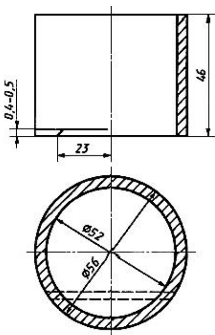
Черт.1. Приспособление для нанесения дисперсии
