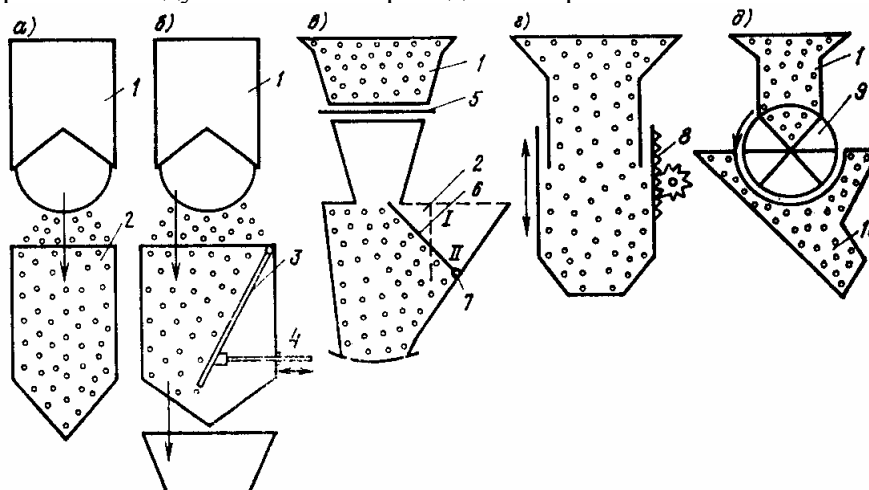
РИС. 6 СХЕМЫ ОБЪЕМНО-ВЕСОВЫХ ДОЗАТОРОВ (по данным ВНИИжелезобетон)
