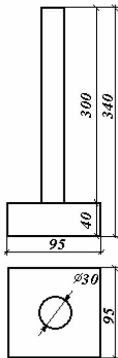
РИС. 5 СТАЛЬНАЯ БОЛВАНКА ДЛЯ ТРАМБОВАНИЯ
