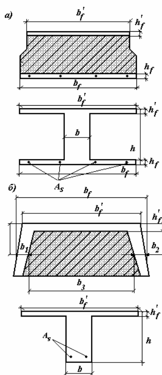
Рис. 4. Схема поперечных сечений составных элементов
